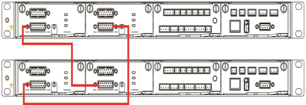
Рис. 3-29. Параллельное кабельное соединение
