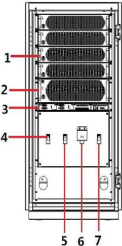
Рис. 2-8. Вид ИБП мощностью 100 кВА спереди (с открытой дверцей)
