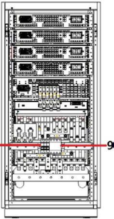
Рис. 2-8. Вид ИБП мощностью 100 кВА спереди (с открытой дверцей)
